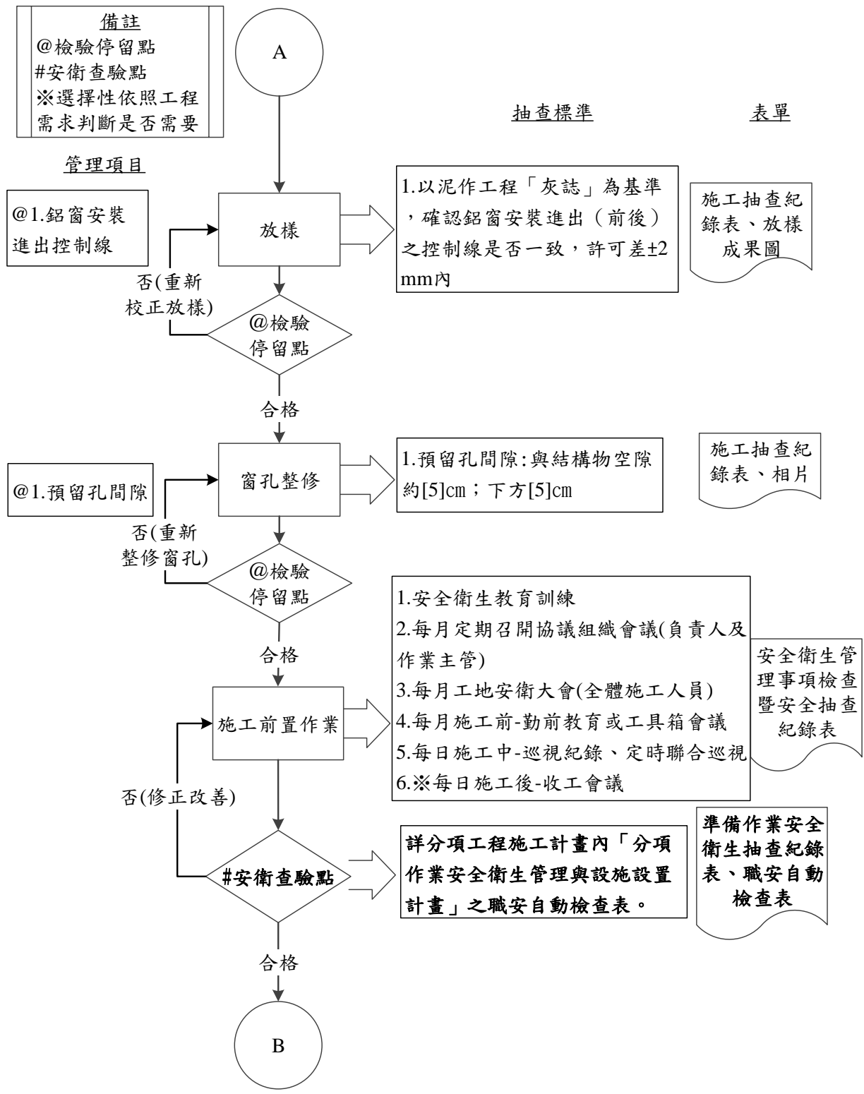
圖 085200-F-1 鋁窗工程施工抽查流程圖 2/4
