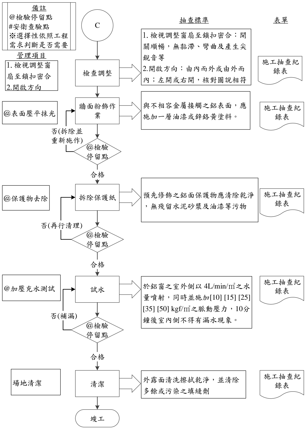
圖 085200-F-1 鋁窗工程施工抽查流程圖 4/4
