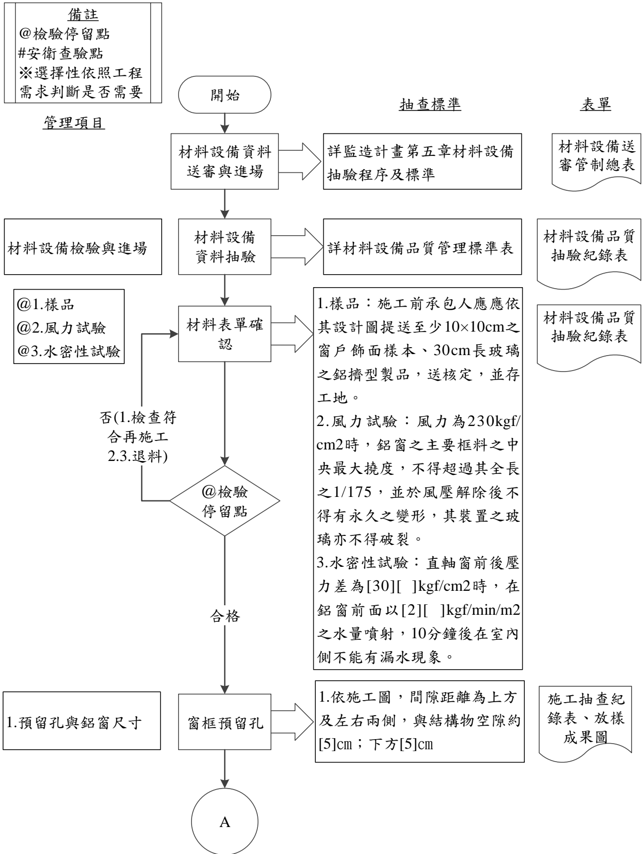
圖 085200-F-1 鋁窗工程施工抽查流程圖 1/4
