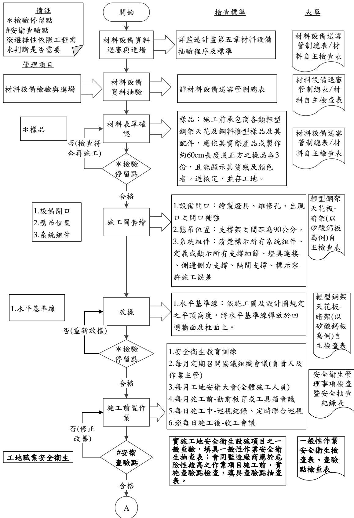
圖 095811-QCF- 1 輕型鋼架天花板-暗架(以矽酸鈣板為例)工程施工流程圖 1/3
