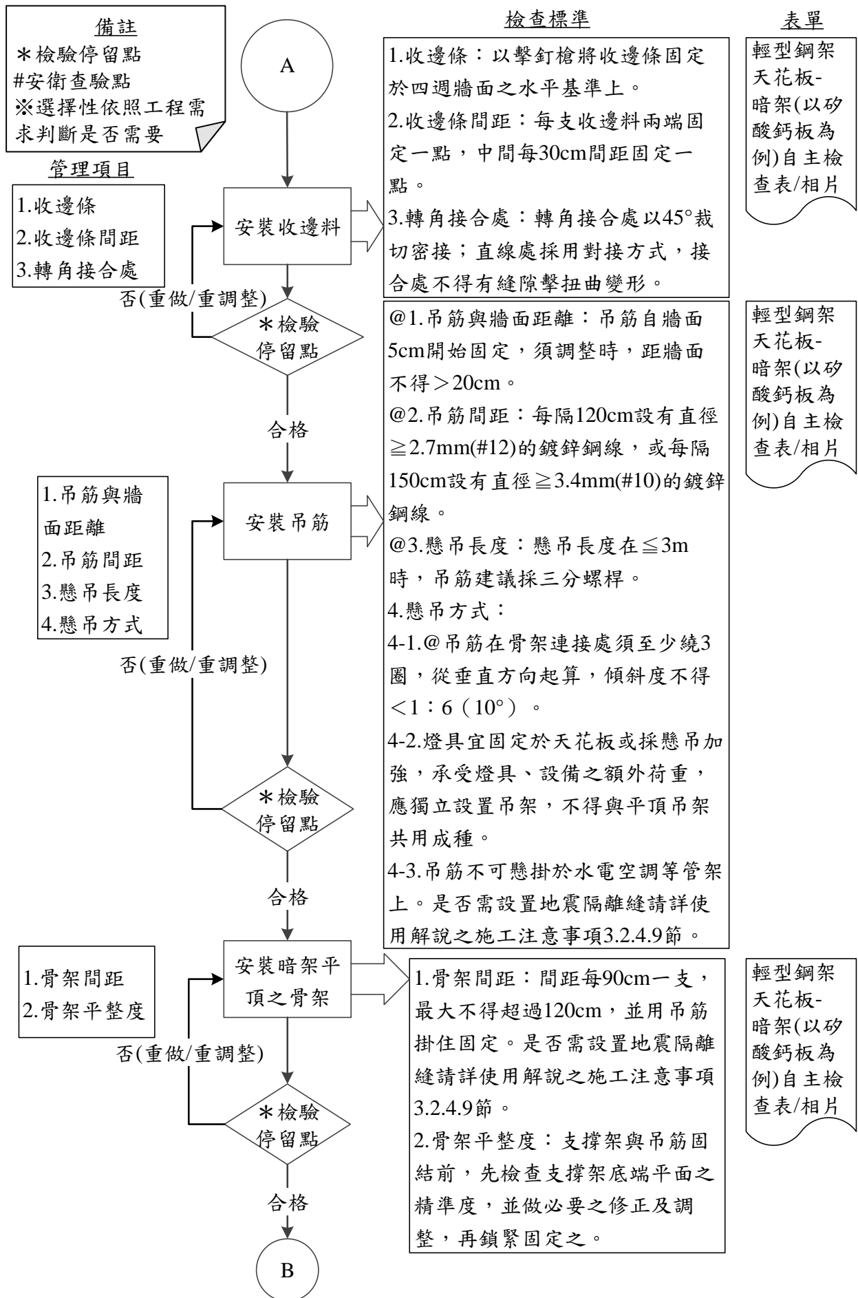
圖 095811-QCF- 2 輕型鋼架天花板-暗架(以矽酸鈣板為例)工程施工流程圖 2/3
