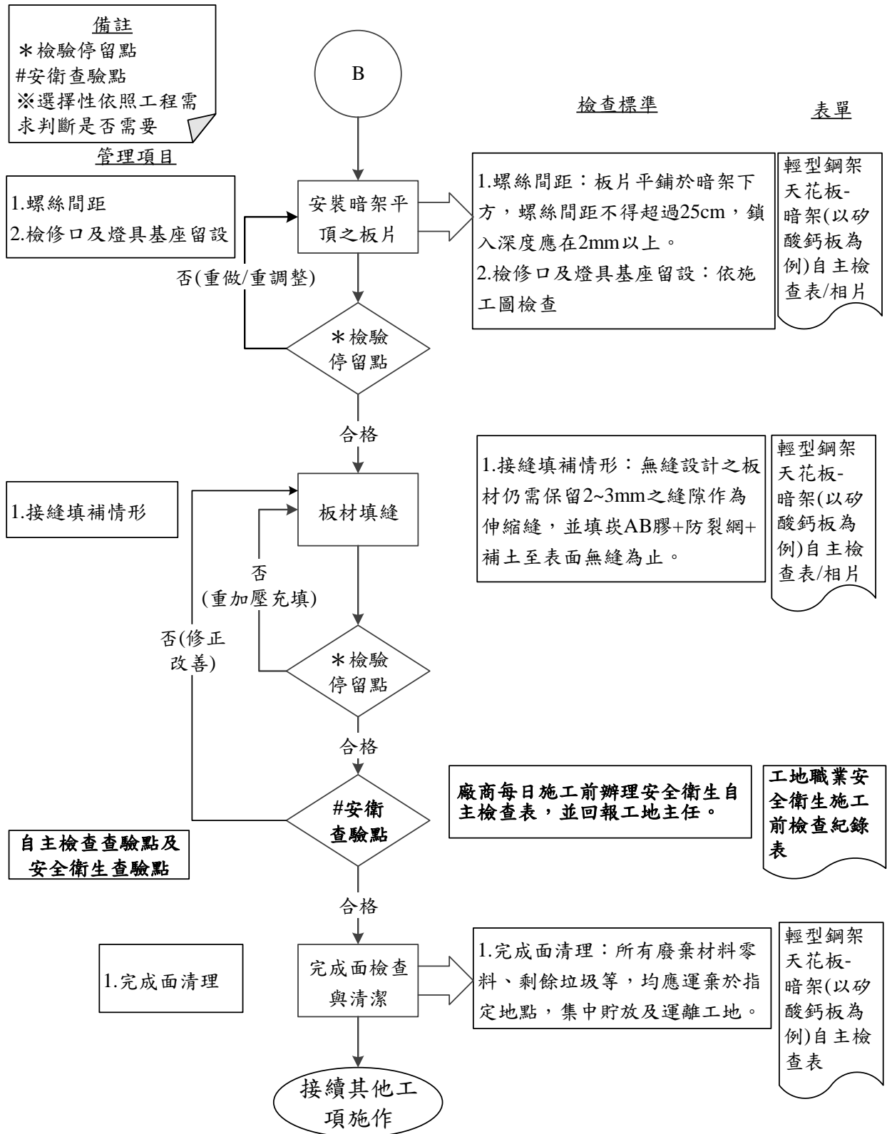
圖 095811-QCF- 3 輕型鋼架天花板-暗架(以矽酸鈣板為例)工程施工流程圖 3/3
