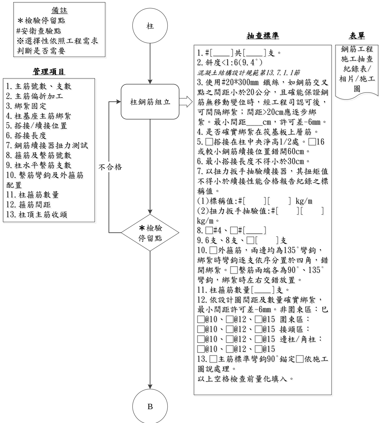
圖 032102-F-1 鋼筋工程施工流程圖 3/7
