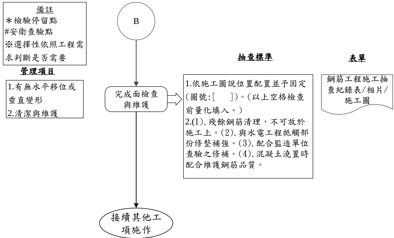
圖 032102-F-1 鋼筋工程施工流程圖 7/7
