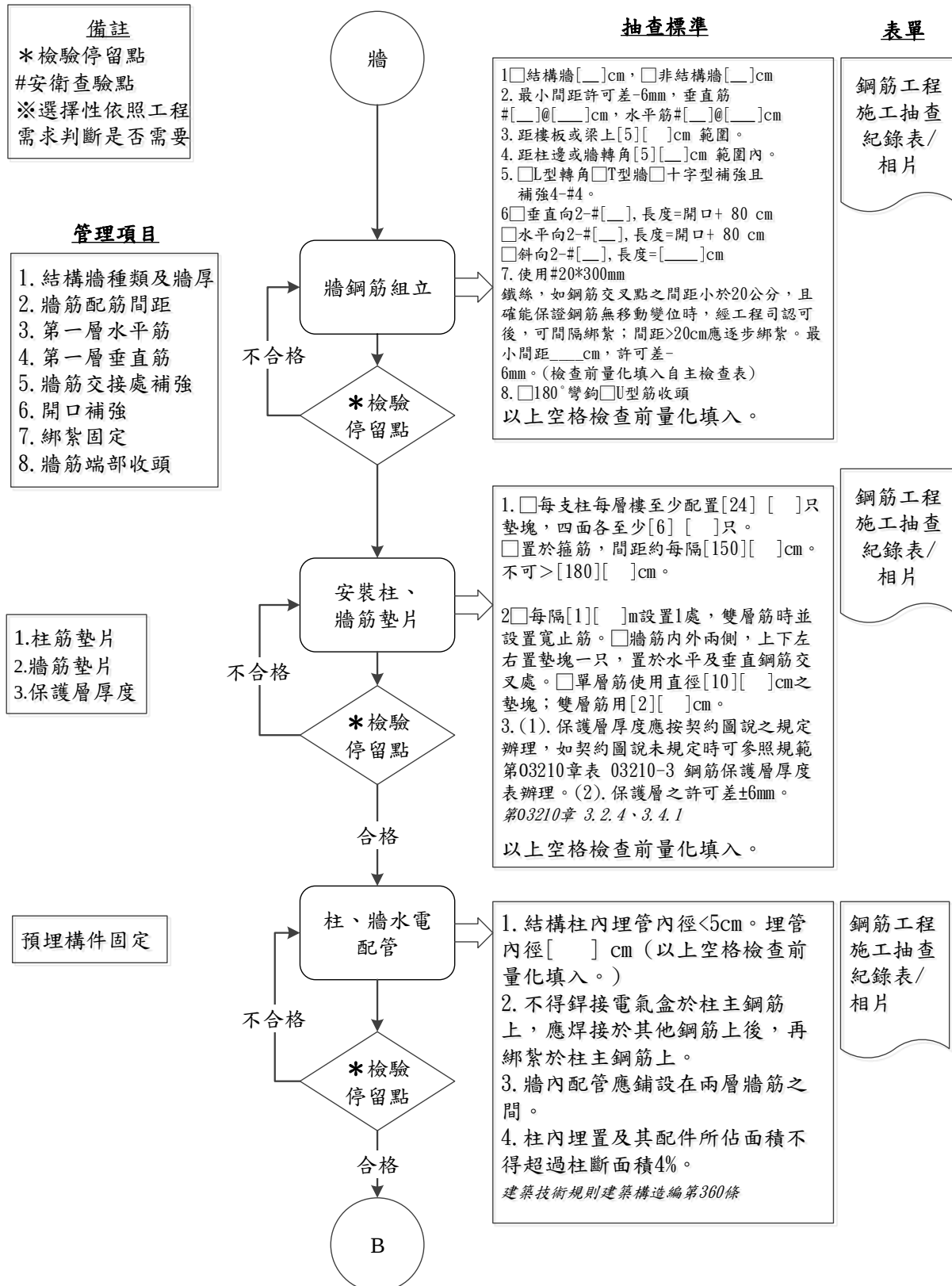
圖 032102-F-1 鋼筋工程施工流程圖 4/7
