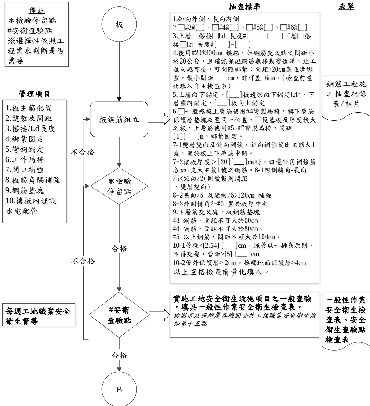
圖 032102-F-1 鋼筋工程施工流程圖 6/7
