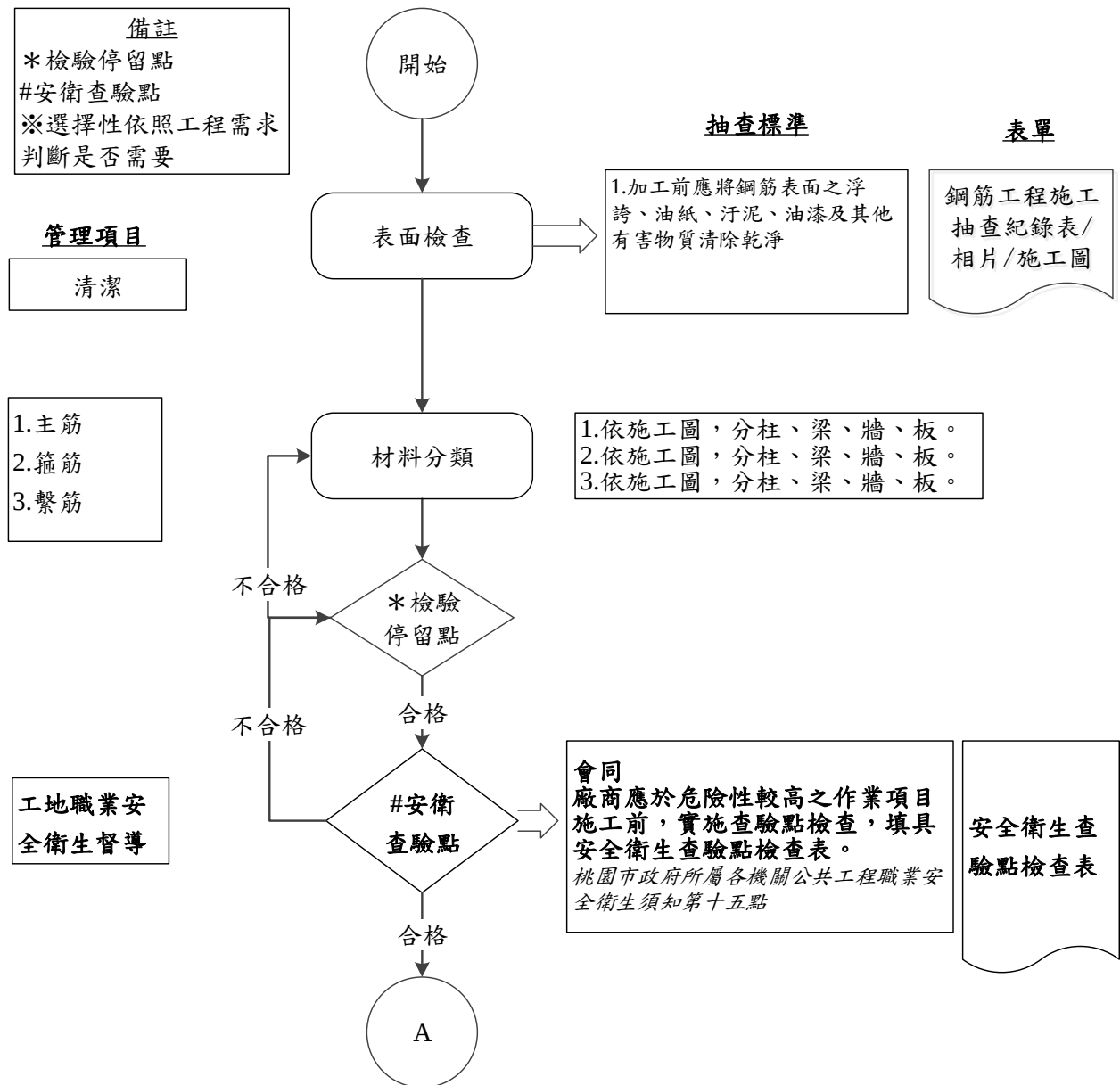
圖 032102-F-1 鋼筋工程施工流程圖 1/7
