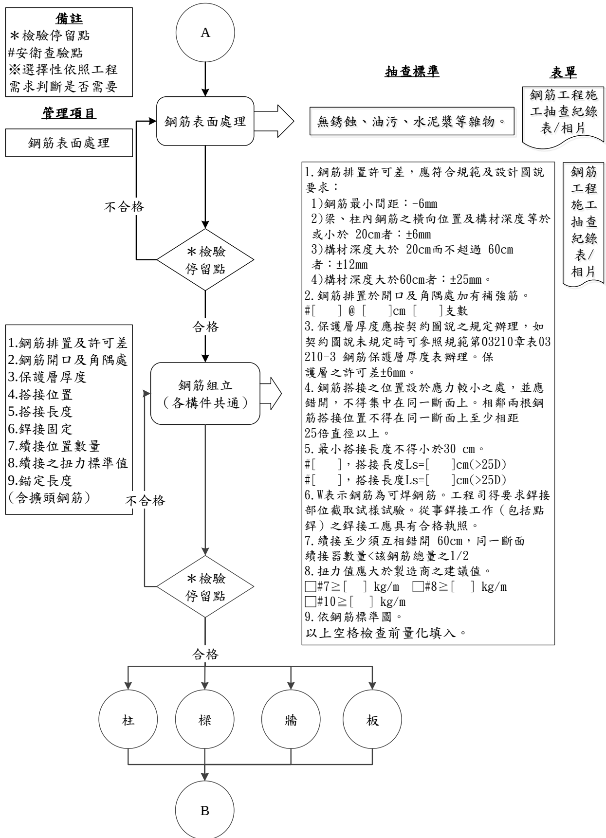
圖 032102-F-1 鋼筋工程施工流程圖 2/7
