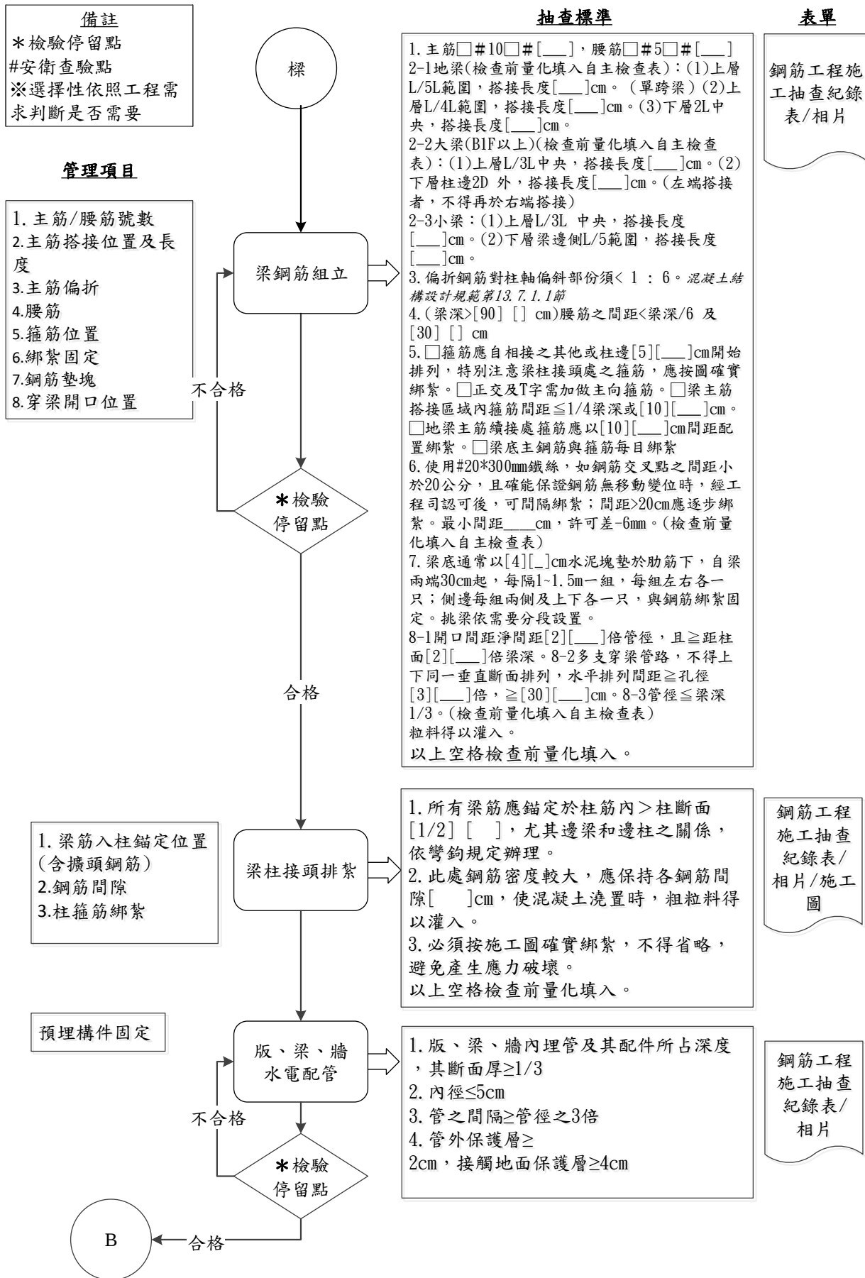
圖 032102-F-1 鋼筋工程施工流程圖 5/7
