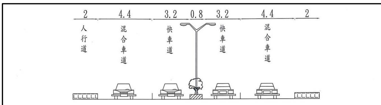
圖 2、車道斷面規劃圖
