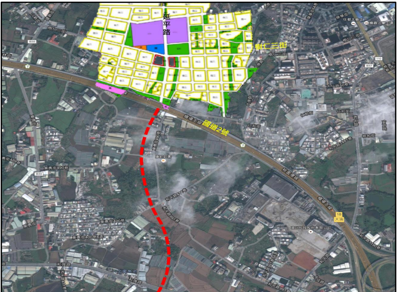
圖 1、延平路(國道 2 號南側)延伸至和平路道路新闢工程(國道 2 號至和強路) (非都市土地範圍)計畫路線示意圖
