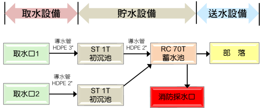
佳志簡水系統供水流程示意圖
