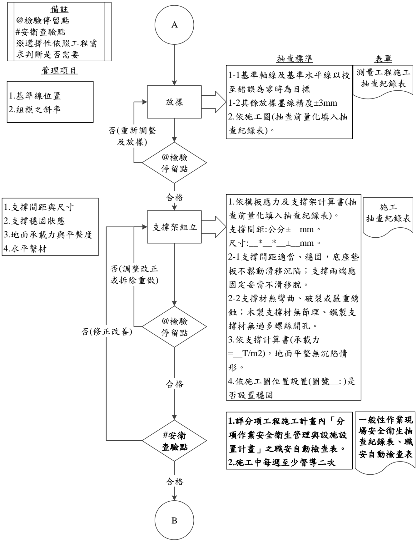
圖 031101-F-1 建築物模板工程施工抽查流程圖 2/3
