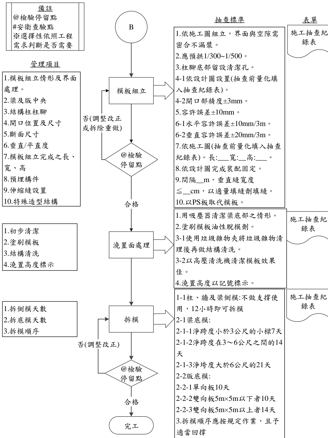
圖 031101-F-1 建築物模板工程施工抽查流程圖 3/3
