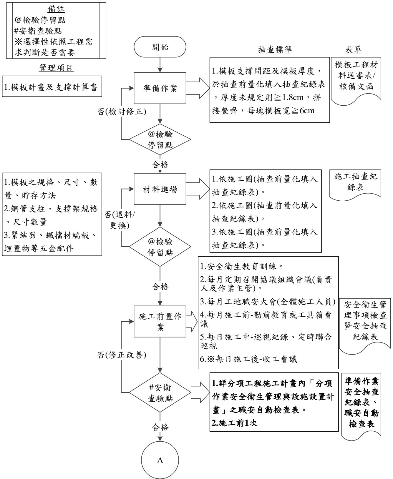
圖 031101-F-1 建築物模板工程施工抽查流程圖 1/3
