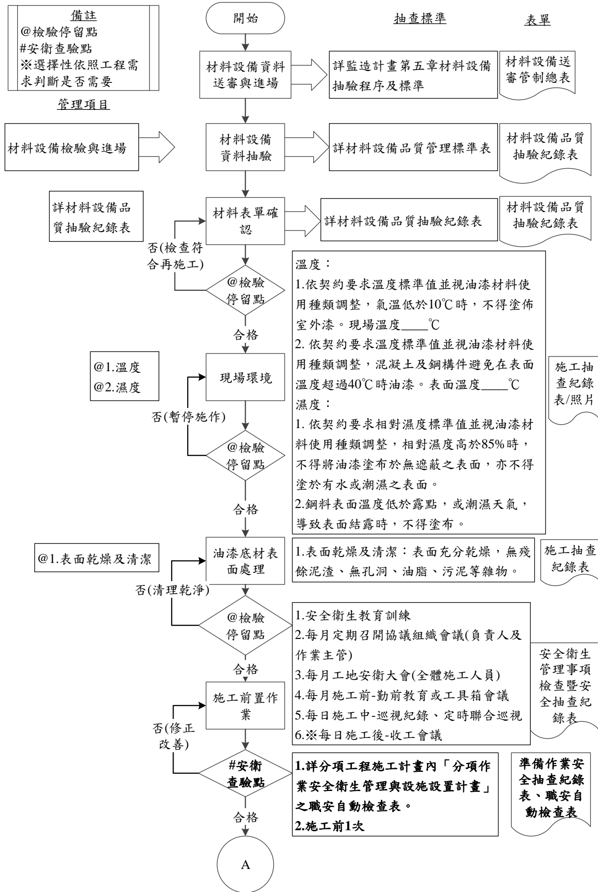
圖 099101-F-1 油漆工程施工抽查流程圖 1/2
