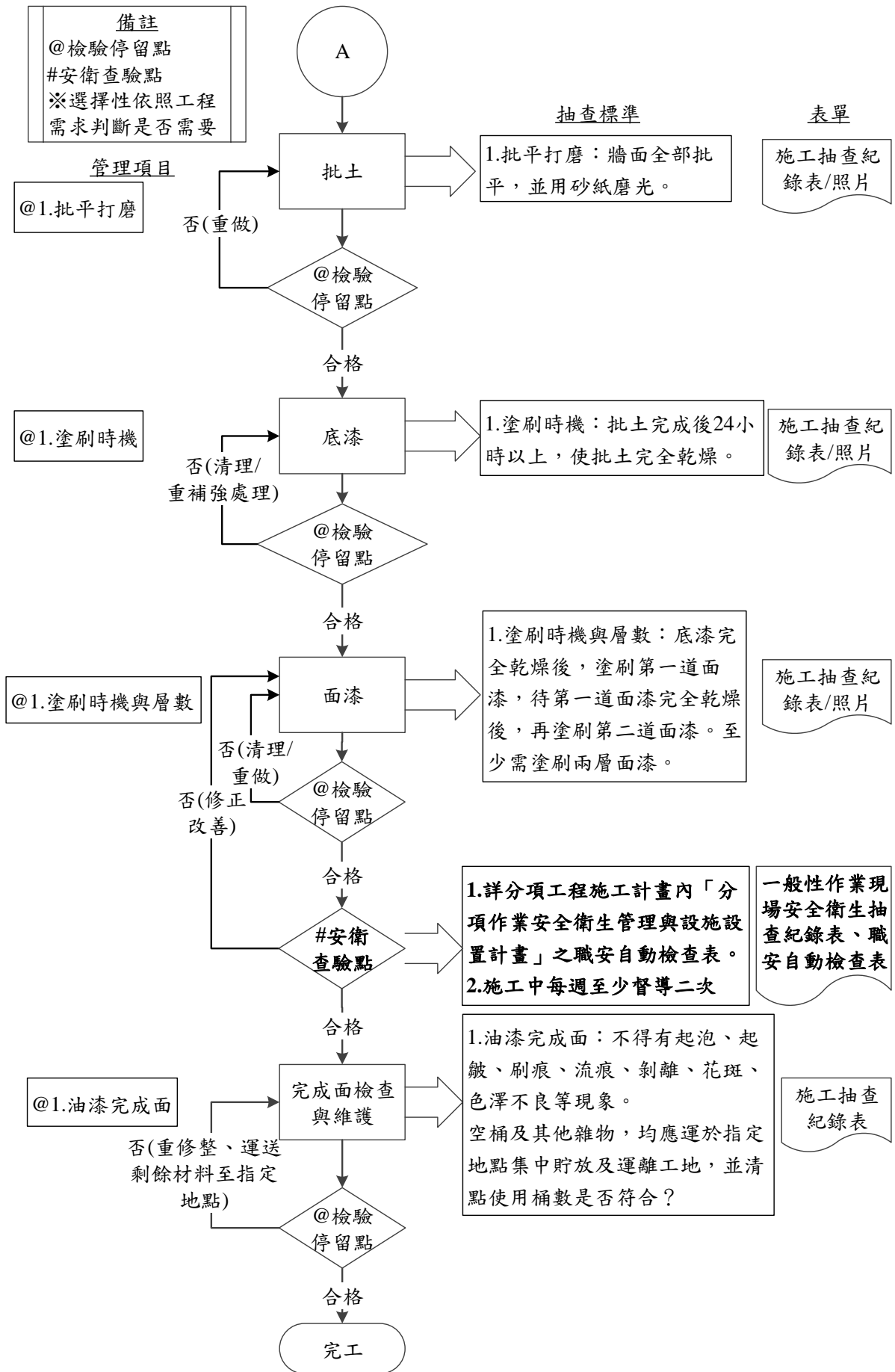
圖 099101-F-1 油漆工程施工抽查流程圖 2/2
