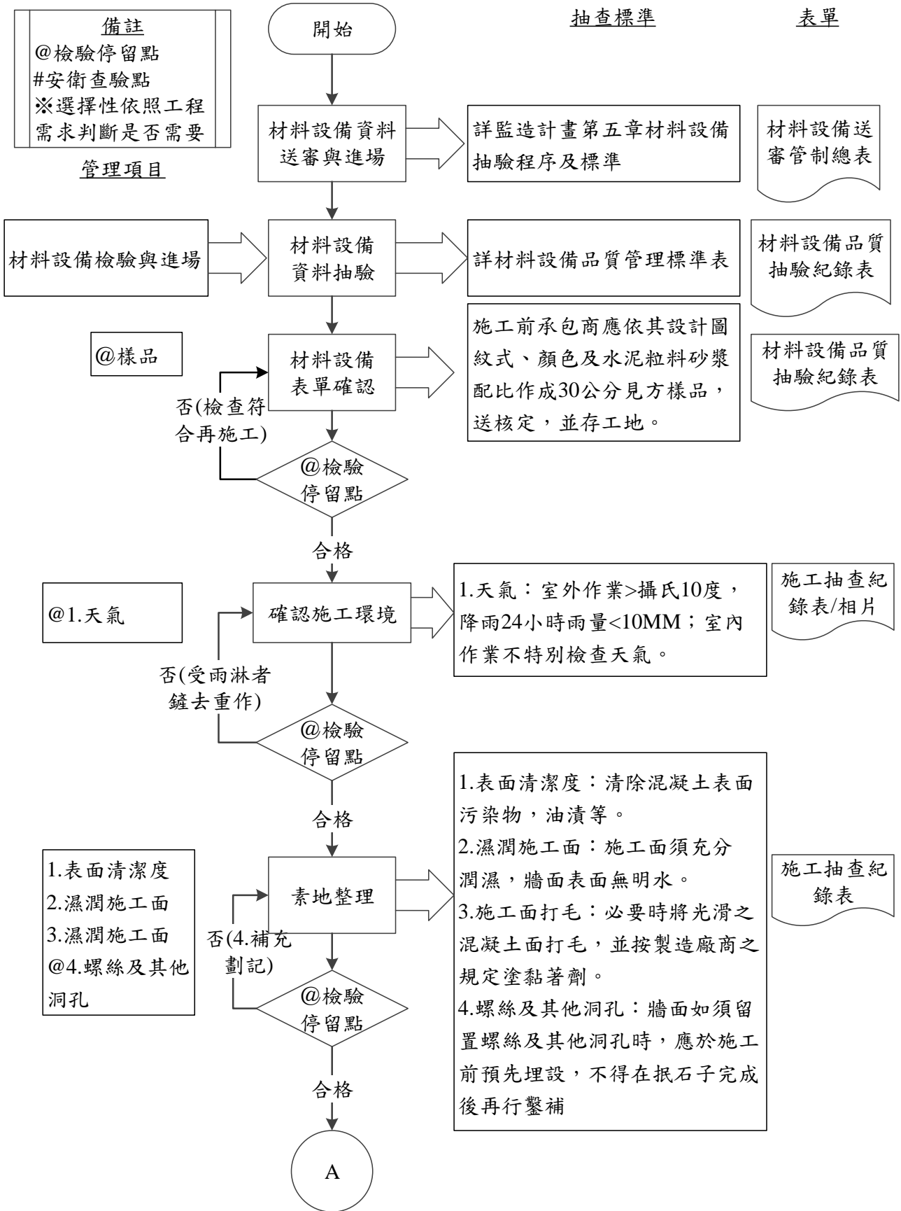
圖 097830-F-1 抵石子工程施工抽查流程图 1/4
