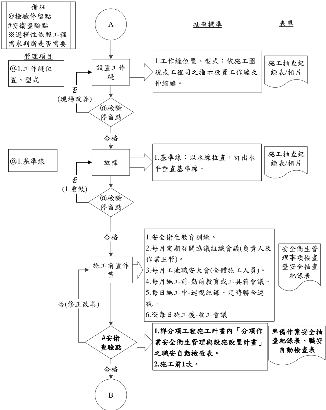
圖 097830-F-1 抵石子工程施工抽查流程圖 2/4
