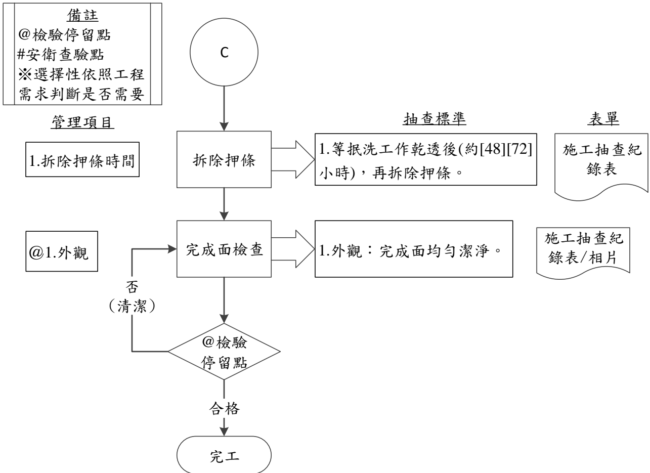
圖 097830-F-1 抵石子工程施工抽查流程圖 4/4
