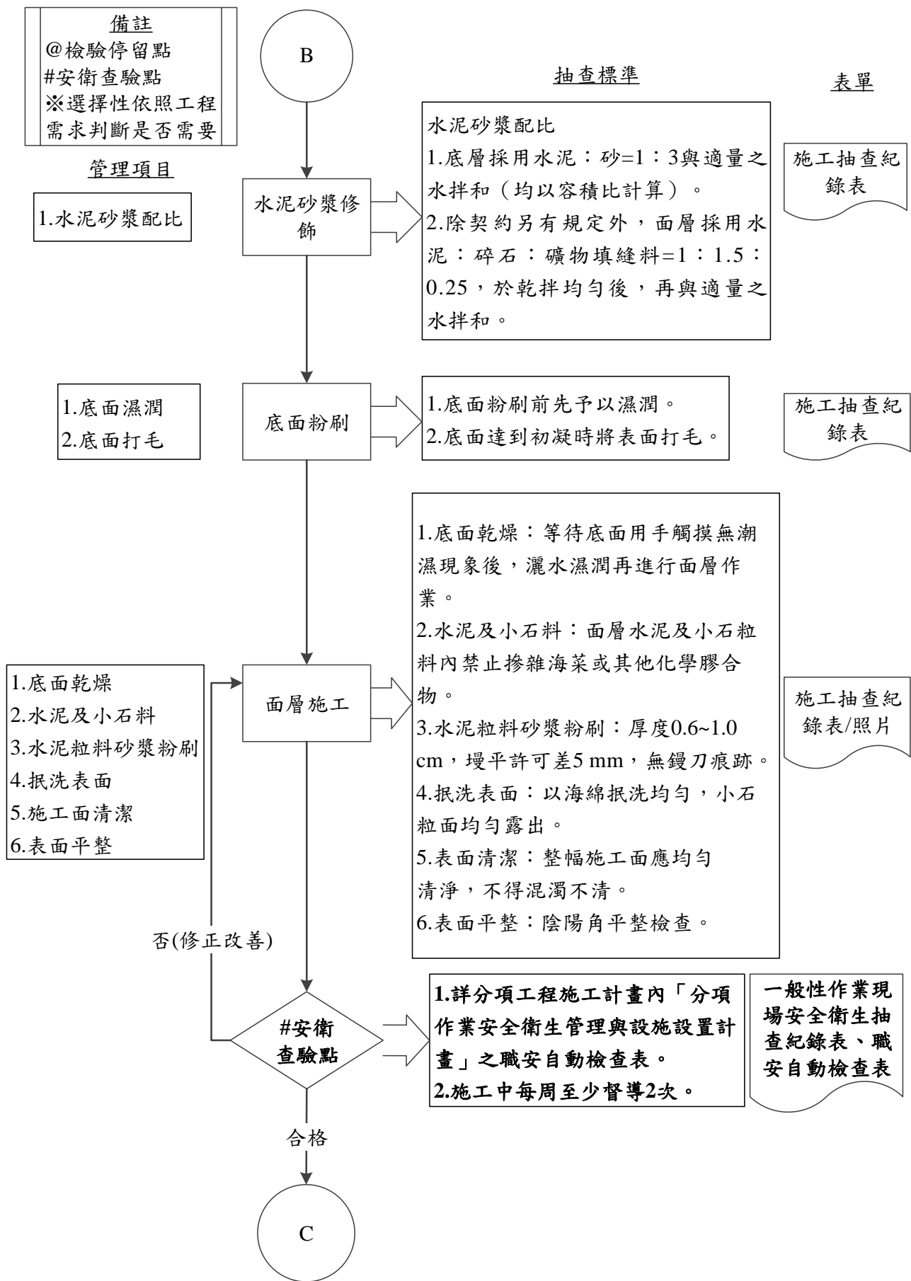
圖 097830-F-1 抵石子工程施工抽查流程圖 3/4
