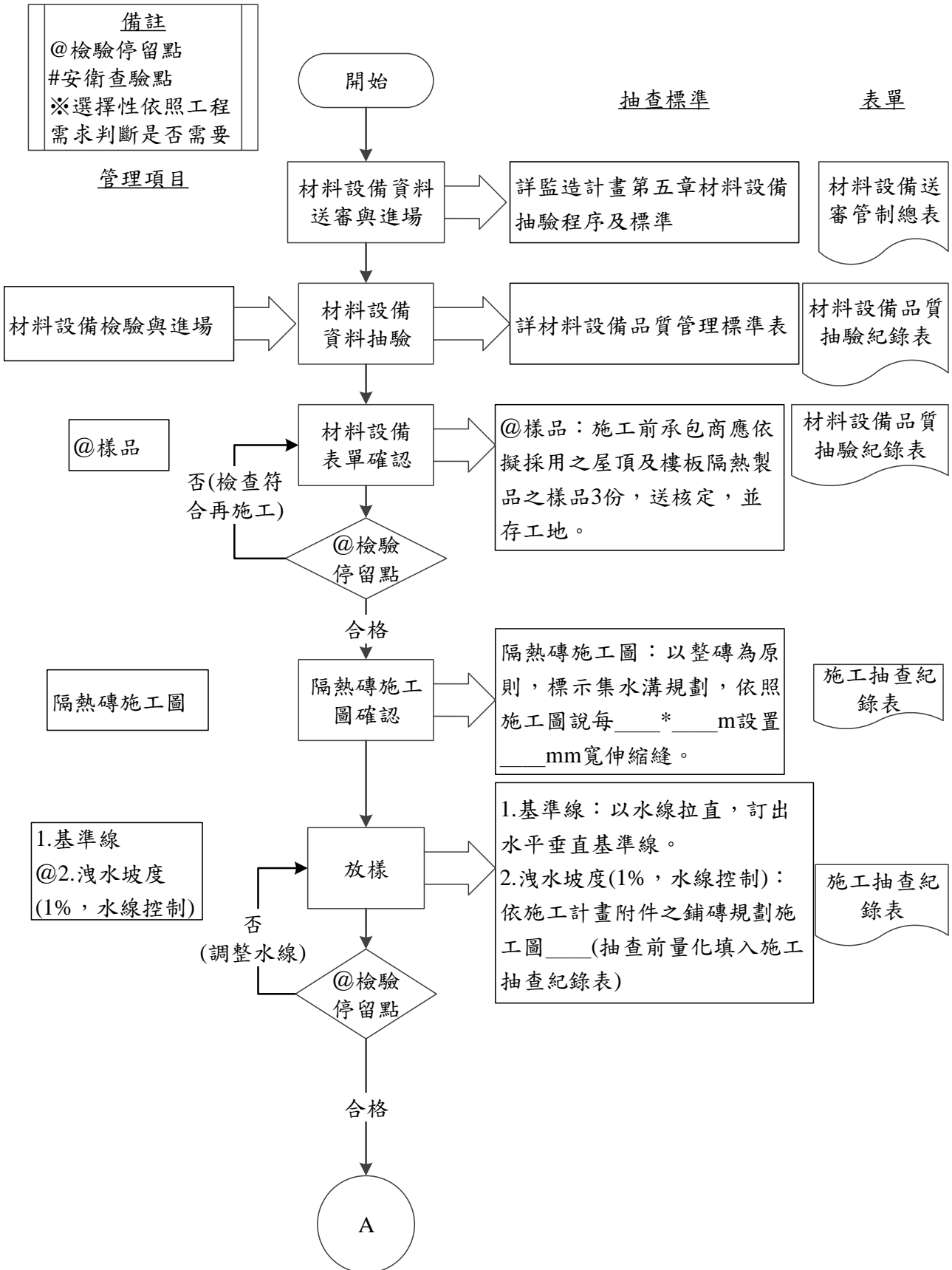
圖 072201-F-1 防水-隔熱磚工程施工抽查流程圖 1/3
