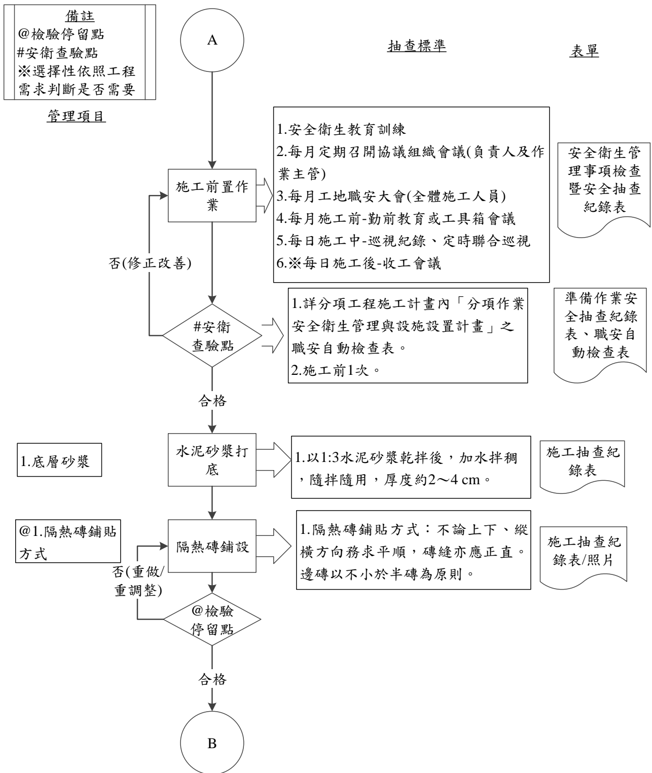
圖 072201-F-1 防水-隔熱磚工程施工抽查流程圖 2/3
