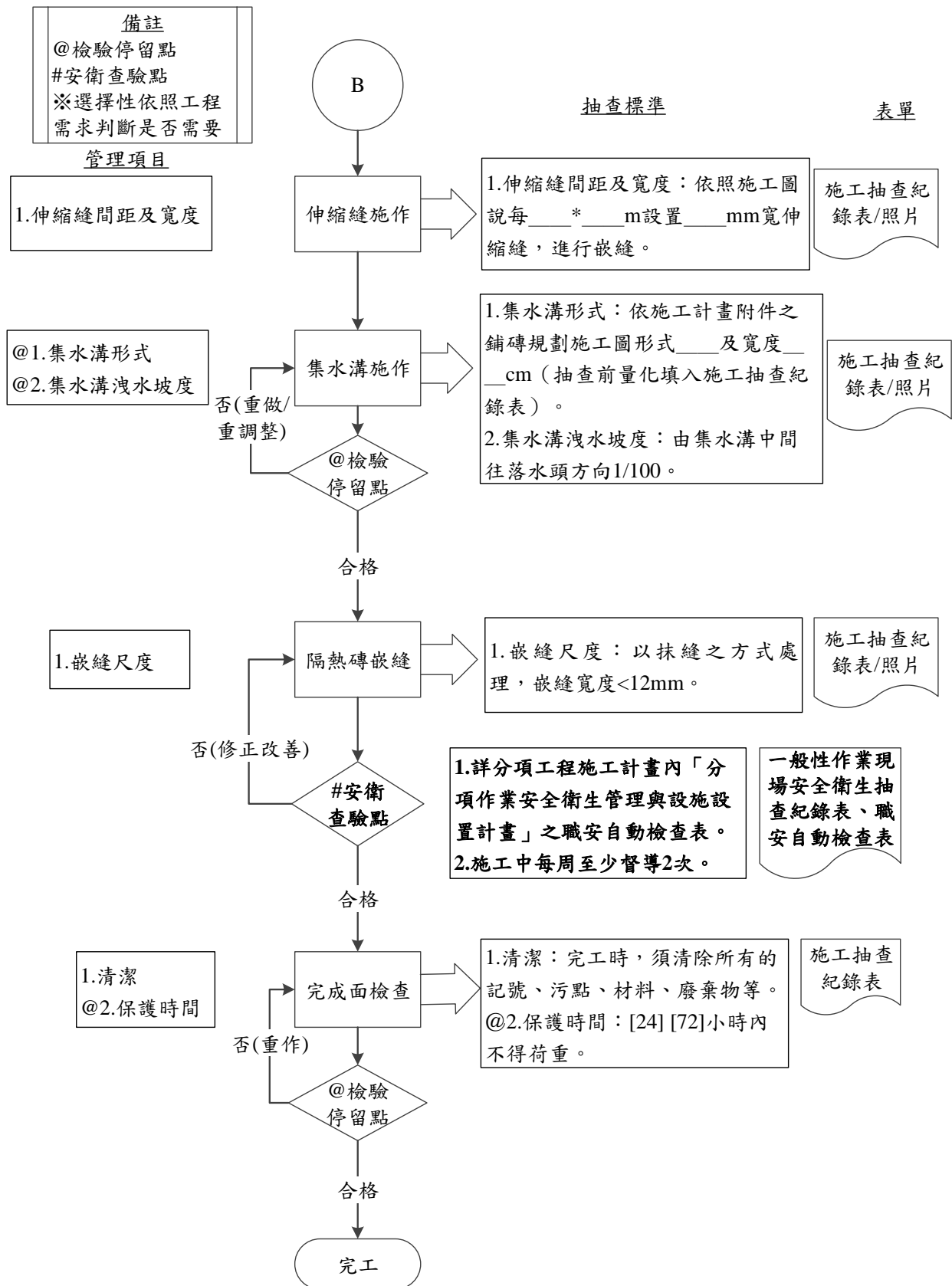
圖 072201-F-1 防水-隔熱磚工程施工抽查流程圖 3/3
