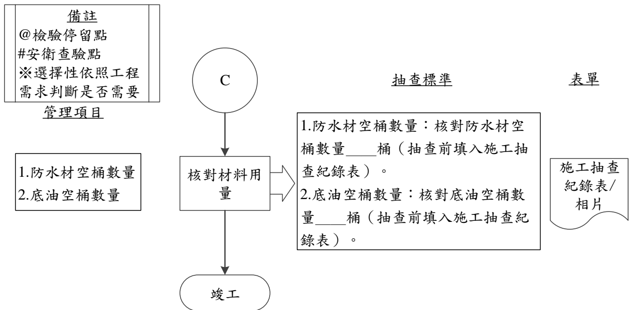
圖 075051-F-1 防水-平屋頂聚胺酯防水膜(PU)工程施工抽查流程圖 4/4
