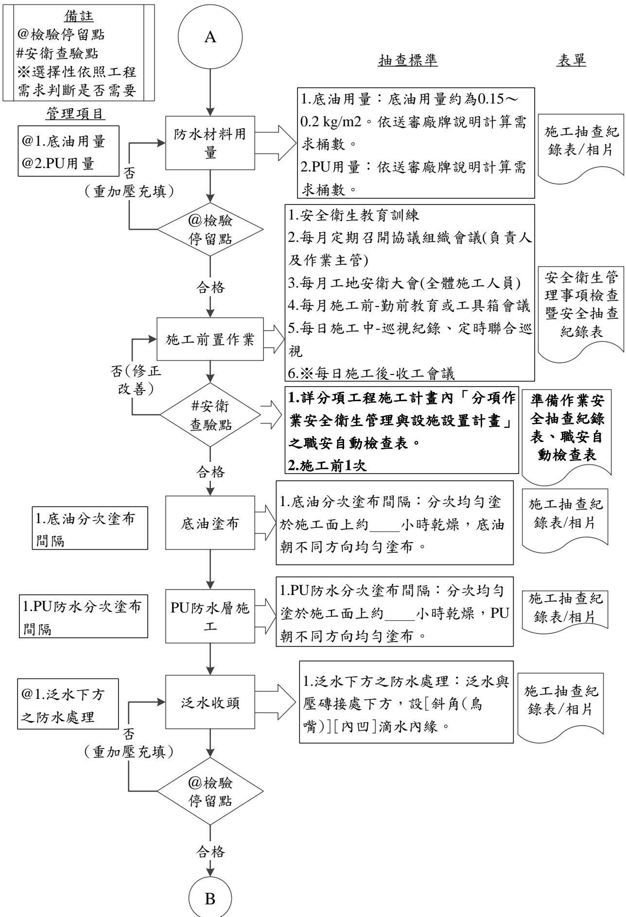
圖 075051-F-1 防水-平屋頂聚胺酯防水膜(PU)工程施工抽查流程圖 2/4
