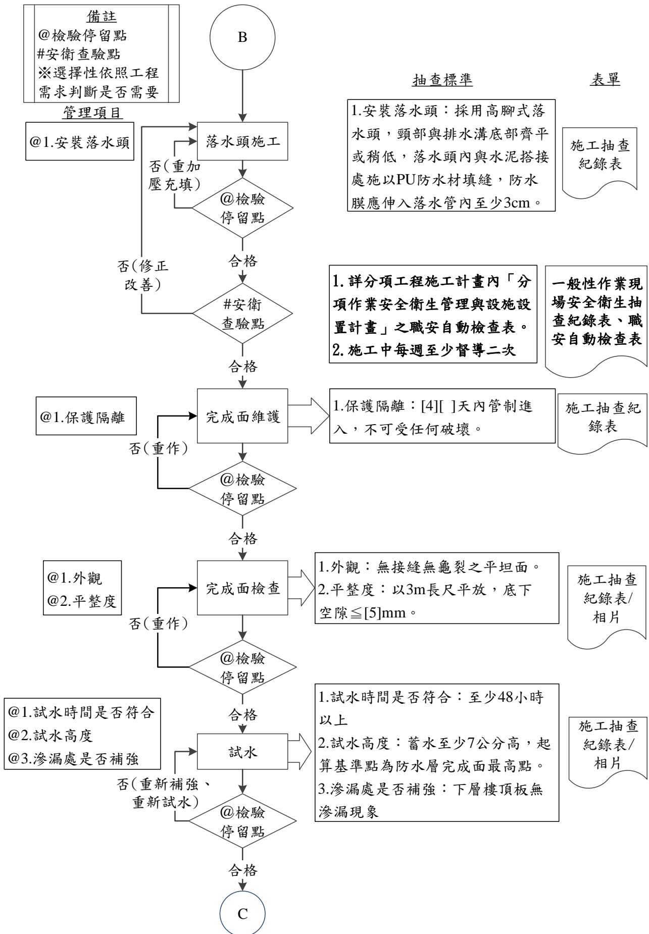
圖 075051-F-1 防水-平屋頂聚胺酯防水膜(PU)工程施工抽查流程圖 3/4
