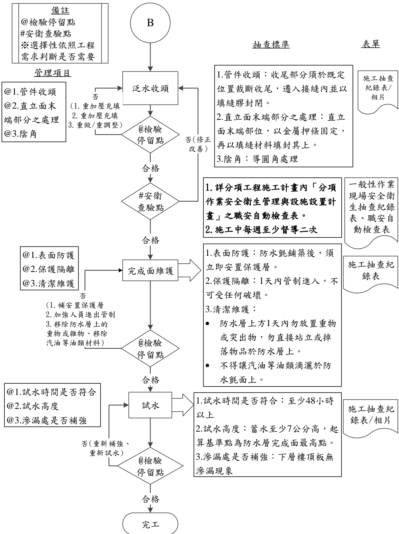
圖 075501-F-1 防水-平屋頂改質瀝青防水氈工程施工抽查流程圖 3/3
