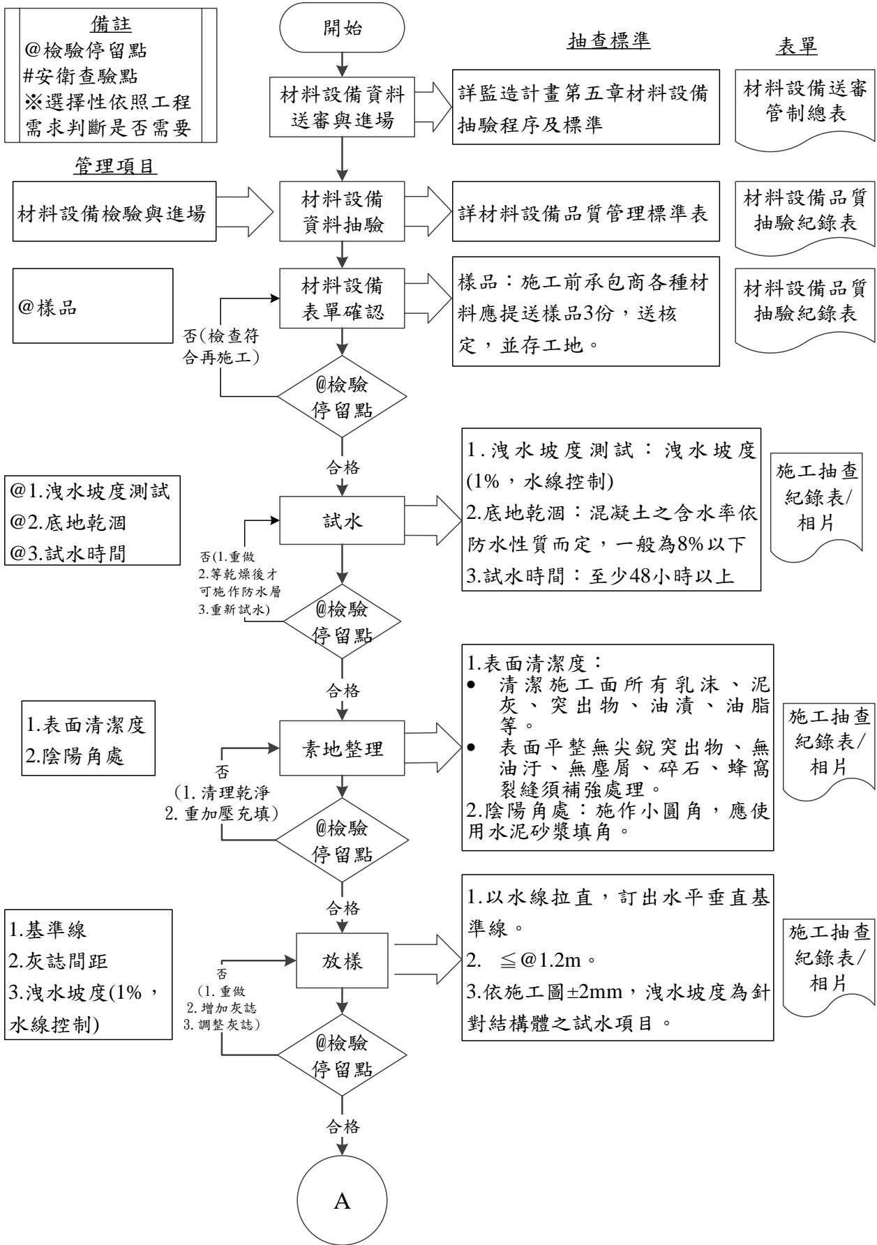
圖 075501-F-1 防水-平屋頂改質瀝青防水氈工程施工抽查流程图 1/3
