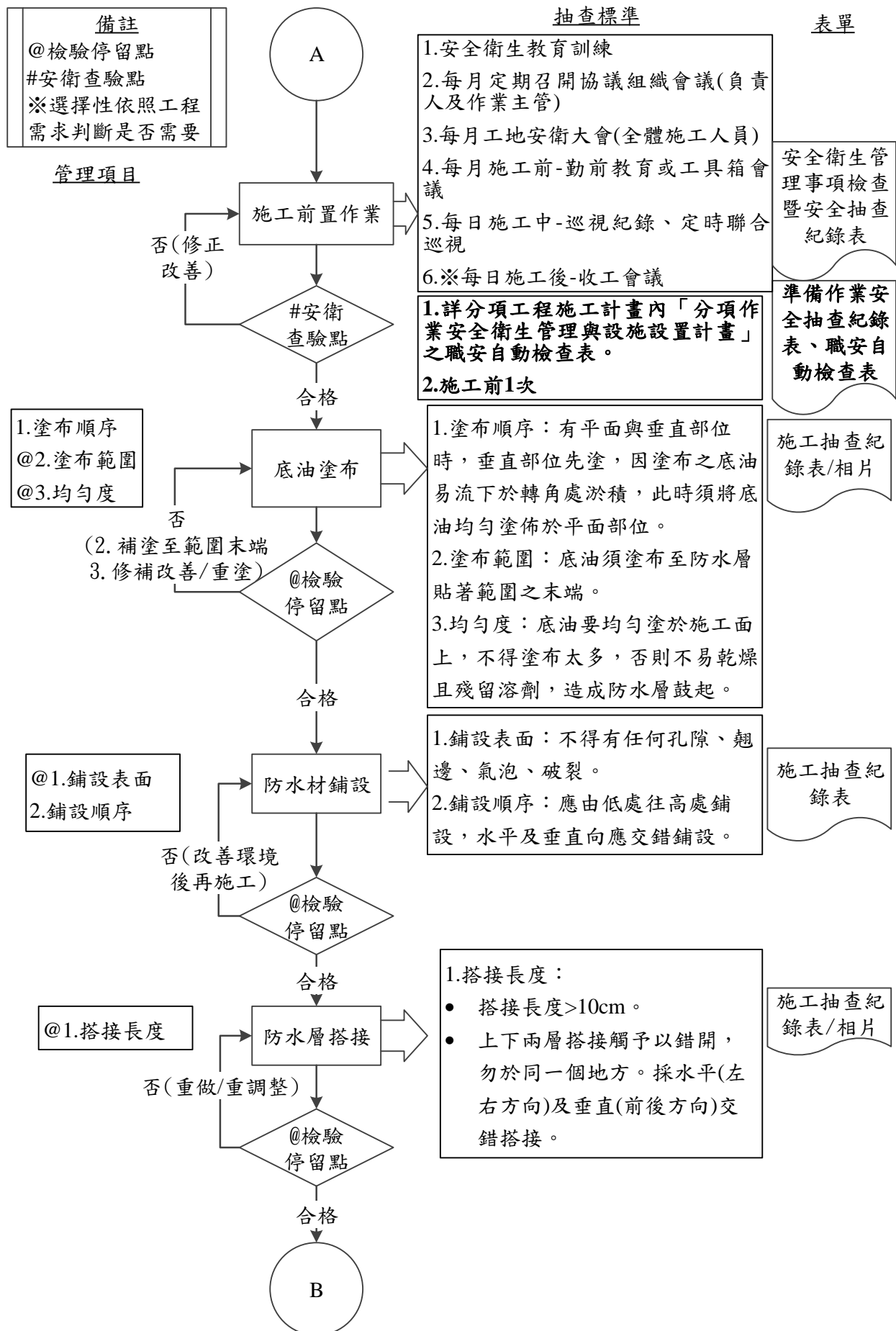
圖 075501-F-1 防水-平屋頂改質瀝青防水氈工程施工抽查流程圖 2/3
