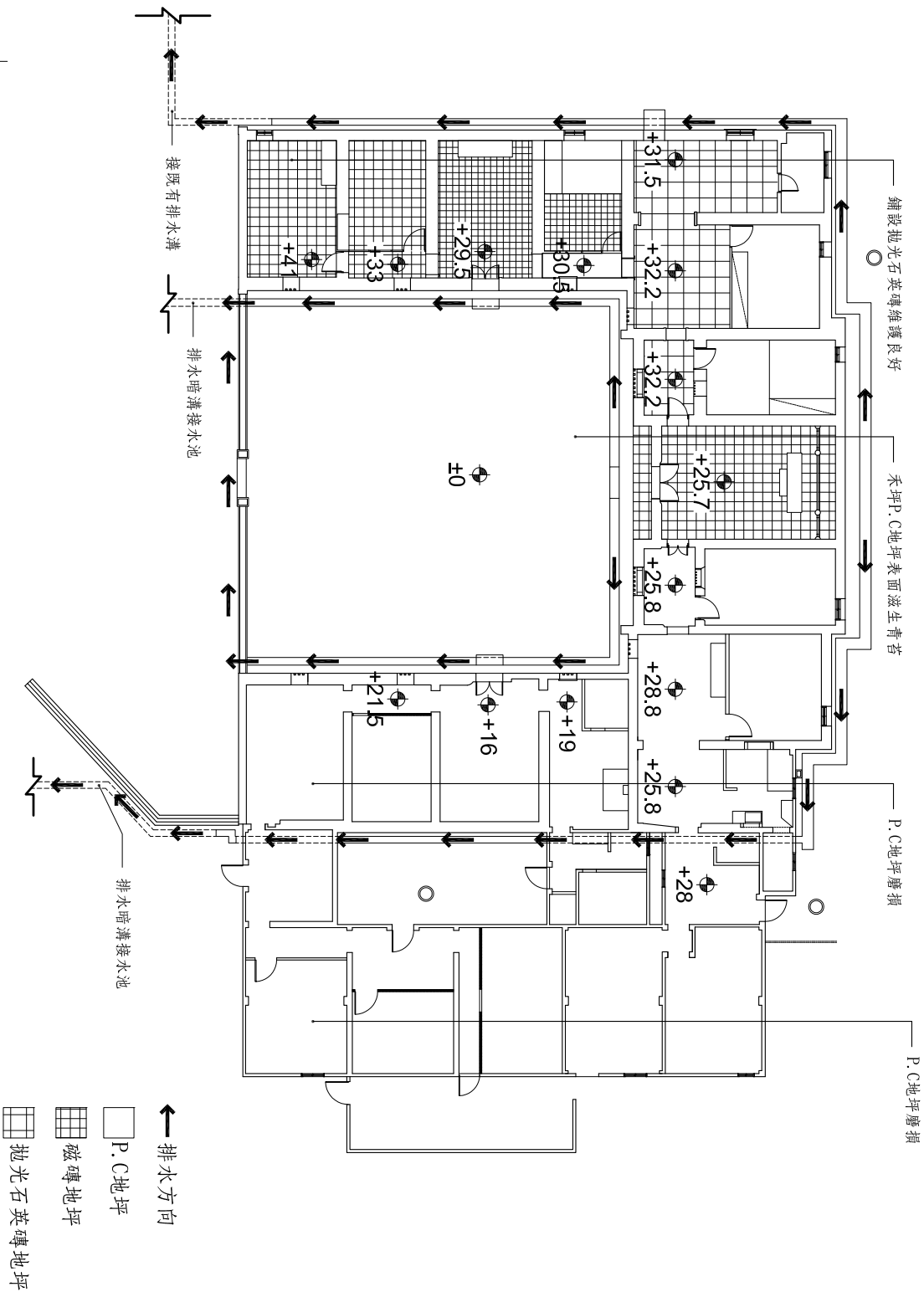
地坪平面圖
