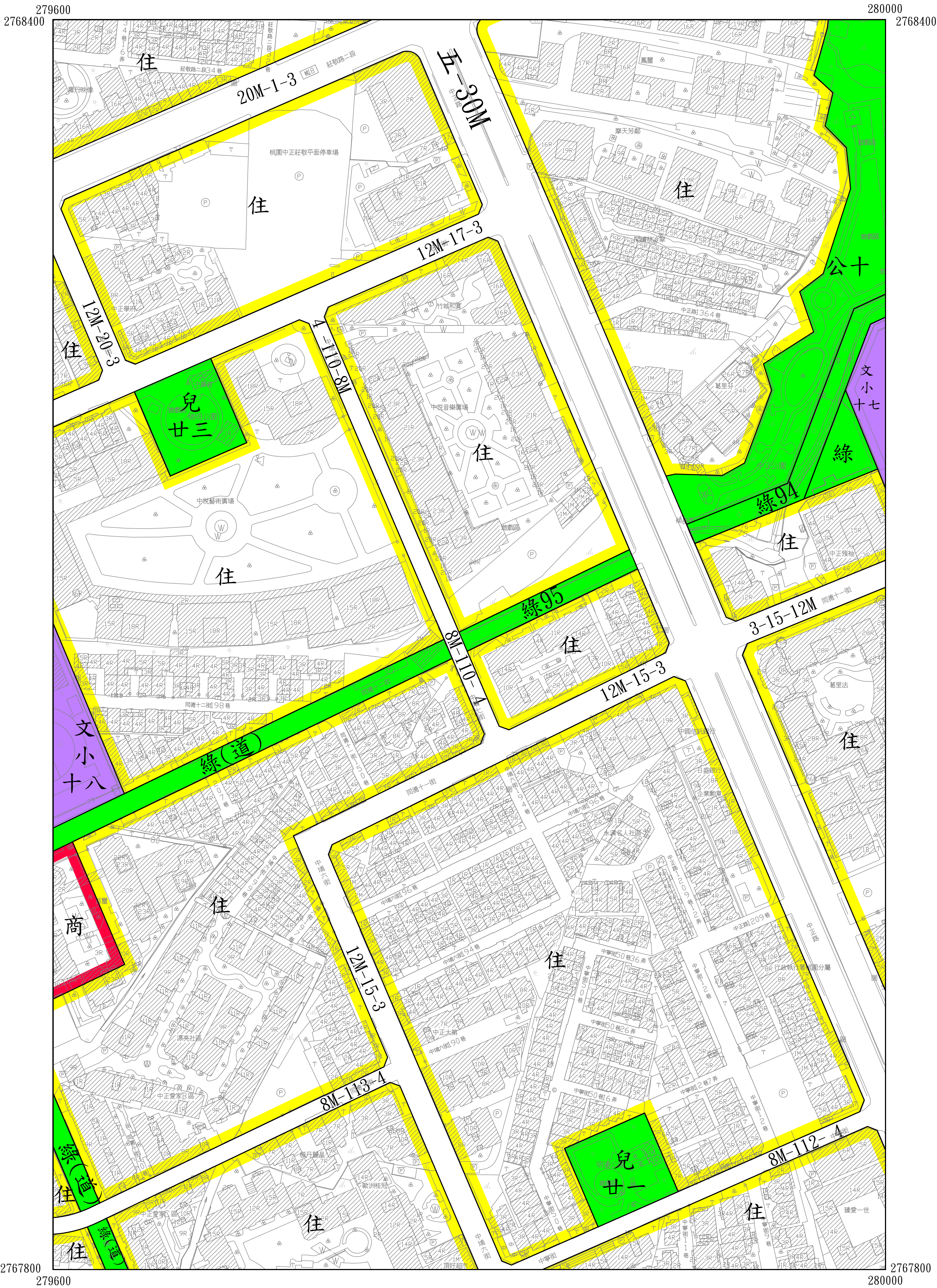
變更南崁地區都市計畫(高速公路南側)細部計畫(第一次通盤檢討)(第一階段)圖
