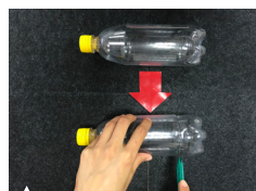
▲ 將寶特瓶距離瓶口12公分處剪開
