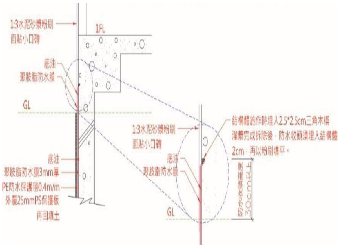
圖 2.1：防水細部圖
