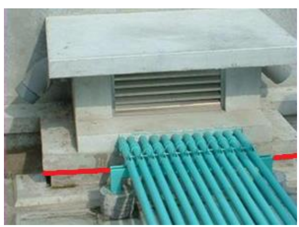
圖8.6：管道間須設泛水
