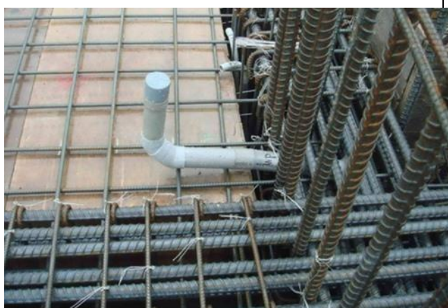
圖 9.1：結構體灌漿前以標高器抓洩水坡度 1/200
