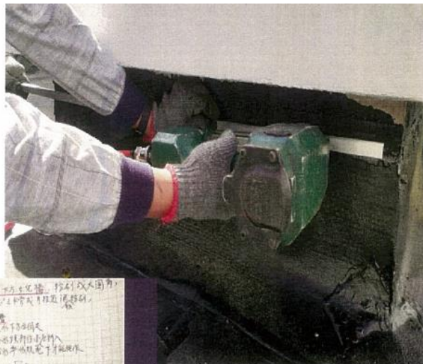
搭接封膠(含壁體 L 型鋁製壓條)
