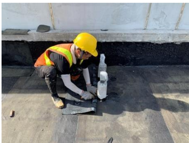
圖 10.5：穿板管開口補強
