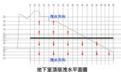
地下室頂版洩水水平面圖
