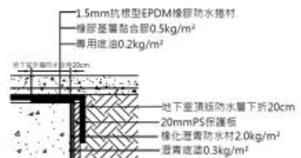
地下外牆防水與地下室頂版防水搭接施工圖
