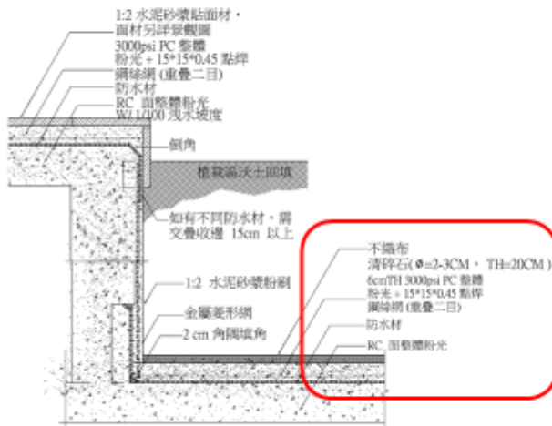
地下室頂版-防水施作詳圖
