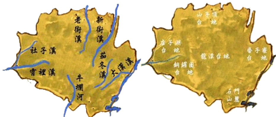
圖0-3、本區河流分布 圖0-4、本區地形分布
