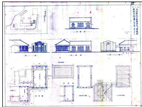
圖 19 1937 年郡役所增建建築圖 資料來源：桃園市文化局，《大溪宿舍群調查研究暨規劃設計擴充案》期末報告書，頁 3-7。
